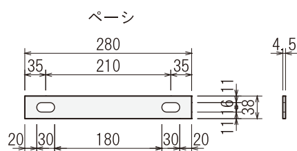
連結金具詳細図
