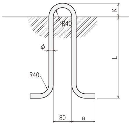
挿入鉄筋図
