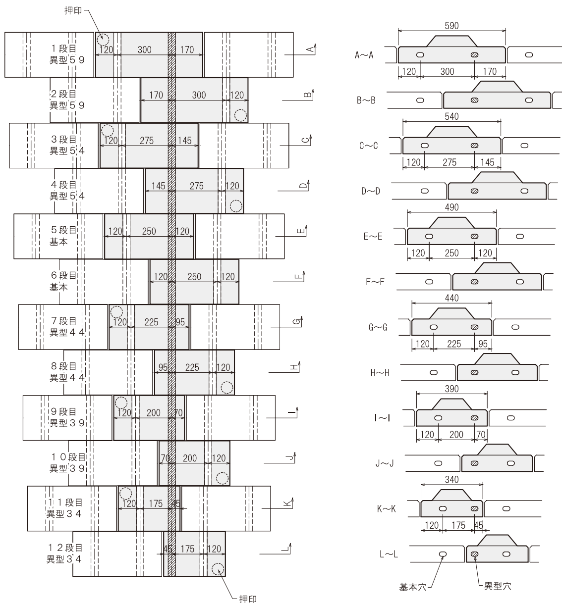
異型ブロック布設詳細図（旭式Y型、旭式A型）
