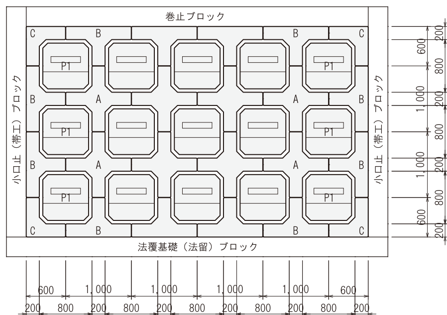
標準布設図
