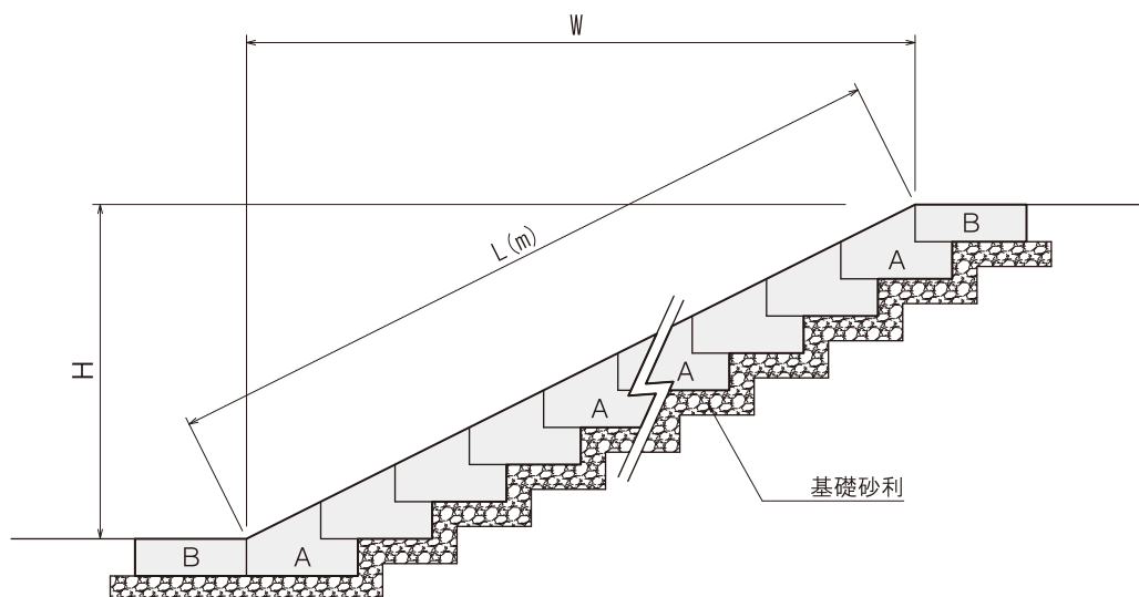
標準断面図
