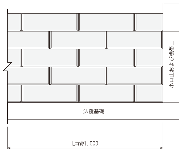
標準布設図
