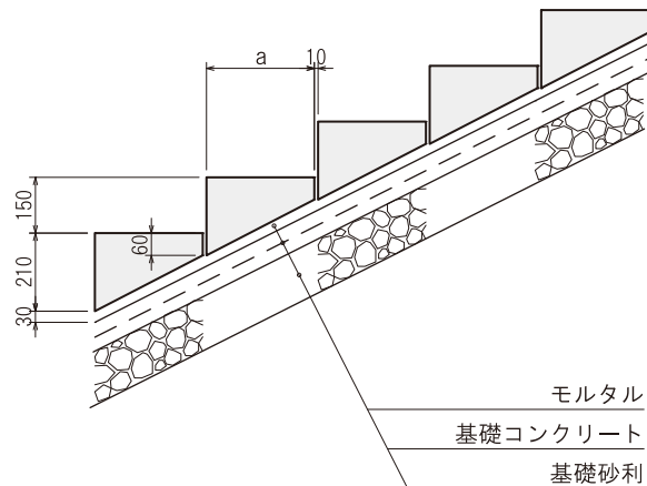
標準断面図
