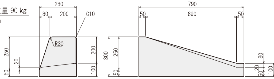
■ 特殊変形 b 質量 49 kg 280×100×790mm
