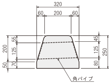
角パイプ詳細図
