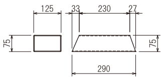
125×75×3.2 溶融亜鉛メッキ (HDZ45)
