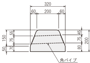
角パイプ詳細図
