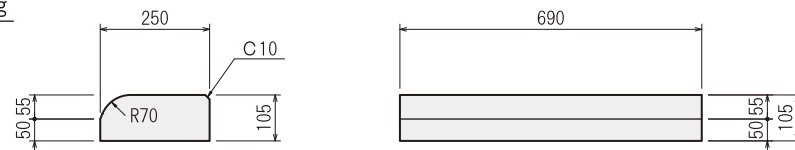
■ 変形 b 質量 41 kg 250×105×690mm
