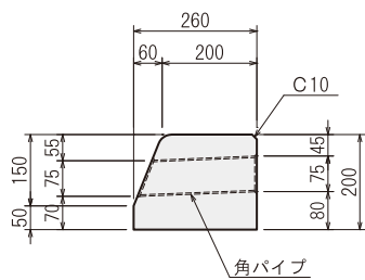
角パイプ詳細図
