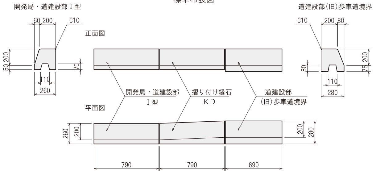
標準布設図
