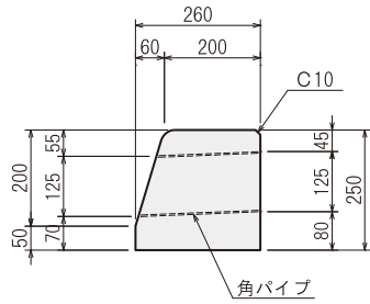
角パイプ詳細図
