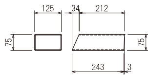
角パイプ詳細図
