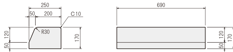
■ 標準 質量 63 kg 250×170×690mm
