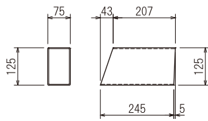
角パイプ詳細図
