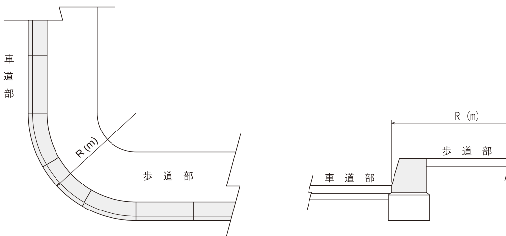
曲線施工時の使用本数(90° 当り)
