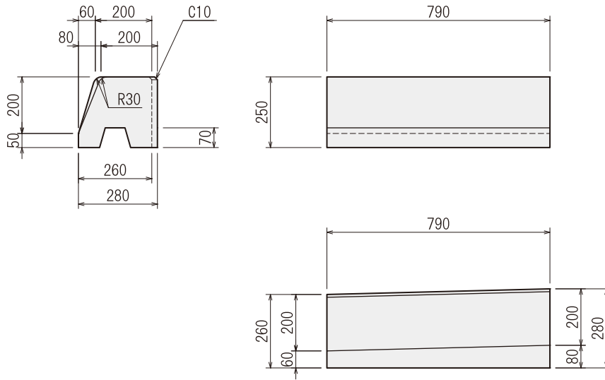
摺付縁石KD 質量98kg
