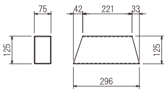
125×75×3.2 溶融亜鉛メッキ (HDZ45)
