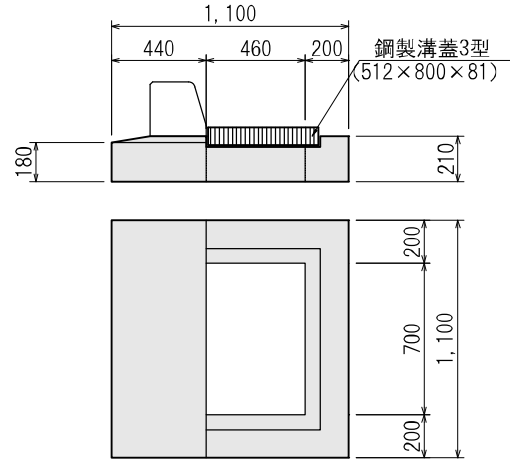
上部 質量 526 kg
