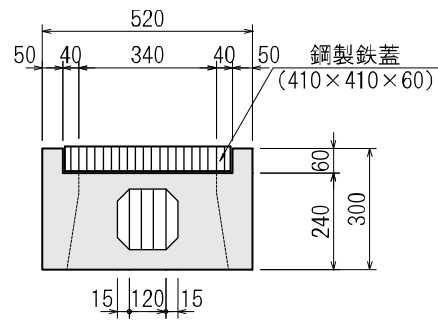
II 型上部
