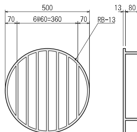
φ450 用
