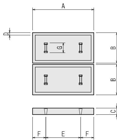
鉄枠コンクリート蓋
