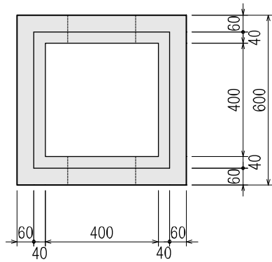
下部 (I・II 共通)
