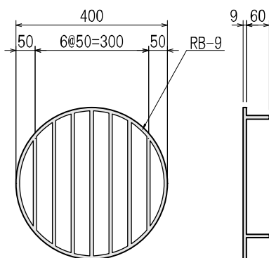
φ350 用
