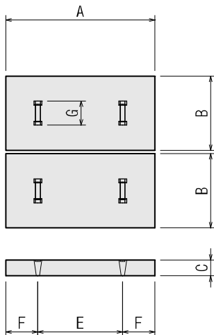
鉄巻コンクリート蓋, コンクリート蓋
