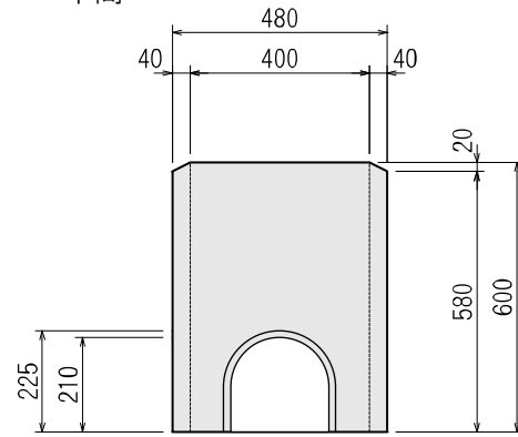
中間
