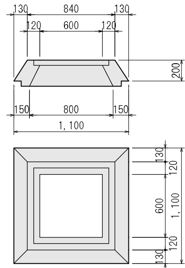
接続柵 質量 263 kg
