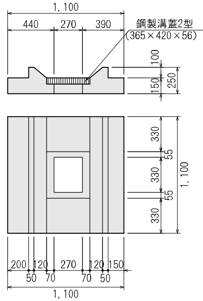
接続柵 質量 263 kg
