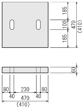
鉄巻コンクリート蓋
