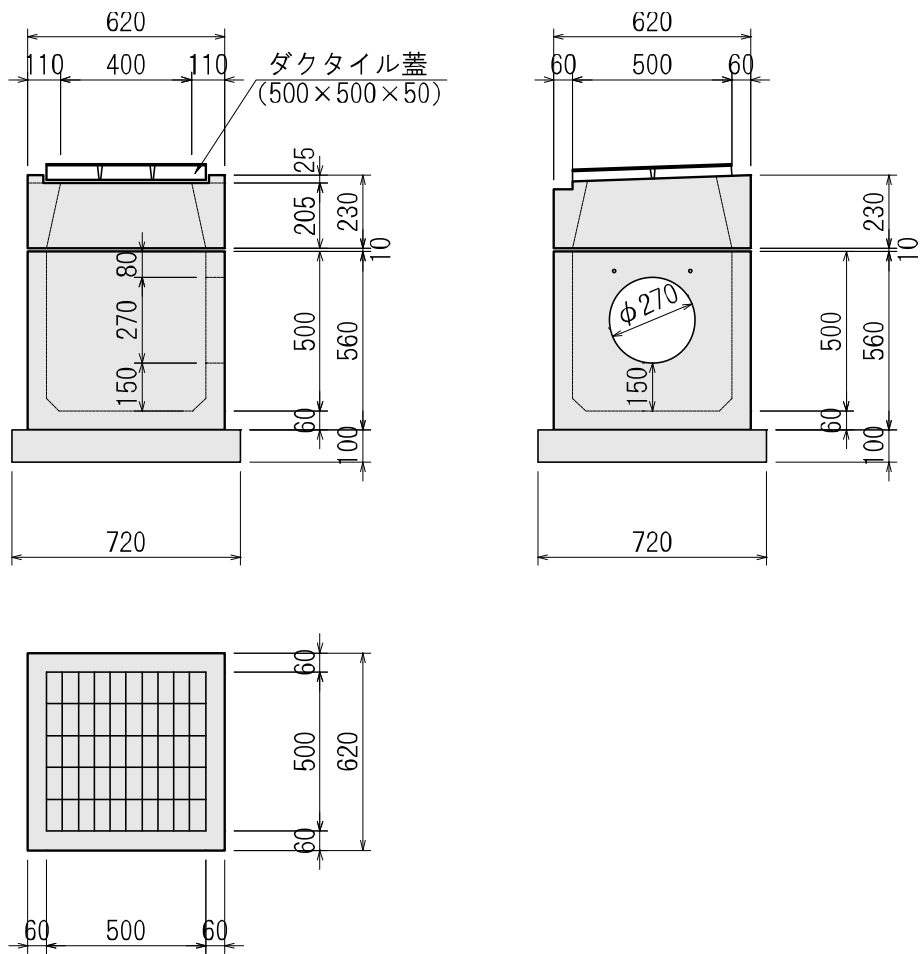
特殊 500 型雨水樹
